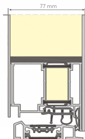
PRZEKRÓJ PRZEZ DRZWI TM 77 HI PRESTIGE - ROZWIĄZANIE PROGOWE
