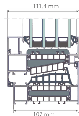
COUPE TRANSVERSALE DE FENÊTRE TM 102HI
