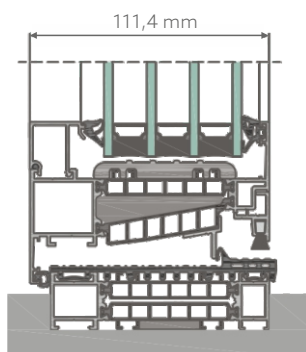
COUPE TRANSVERSALE DE FENÊTRE AU SEUIL BAS TM 102HI
