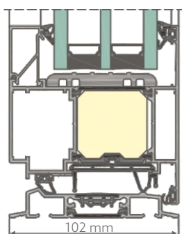
COUPE TRANSVERSALE DE SEUIL DE PORTE
