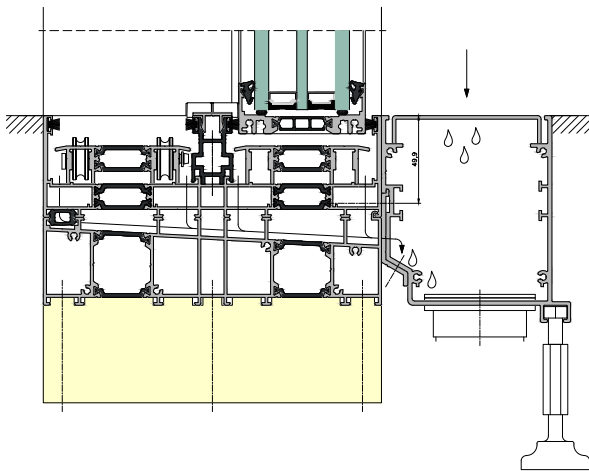
DRAIN LINÉAIRE DANS LE CADRE DU SYSTÈME MOREVIEW
