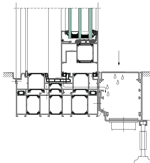
DRAIN LINÉAIRE DANS LE CADRE DU SYSTÈME DP 180
