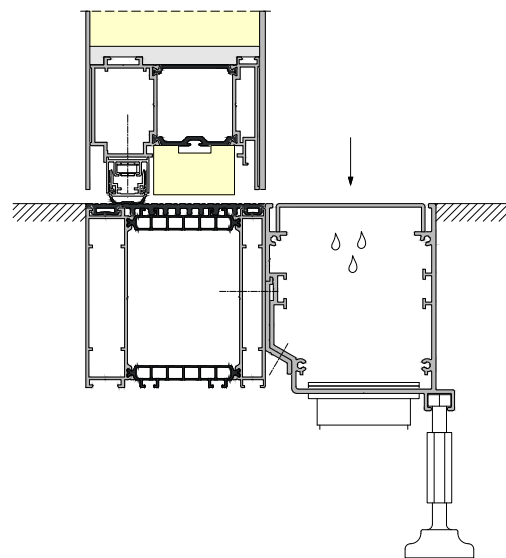
DRAIN LINÉAIRE DANS LE CADRE DU SYSTÈME TM 102HI
